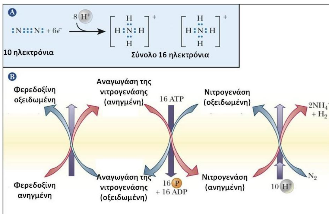
Σχήμα 3.29. Η κατανάλωση ATP κατά την αζωτοδέσμευση και αποτύπωση των χρησιμοποιούμενων ηλεκτρονίων και πρωτονίων κατά την αζωτοδέσμευση.
