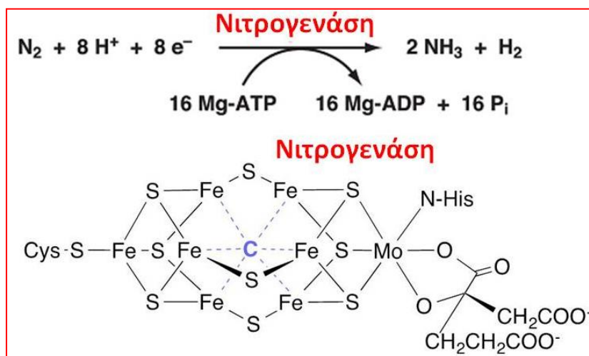
Σχήμα 3.31. Το σύμπλοκο μόριο του ενζύμου νιτρογενάσης.
