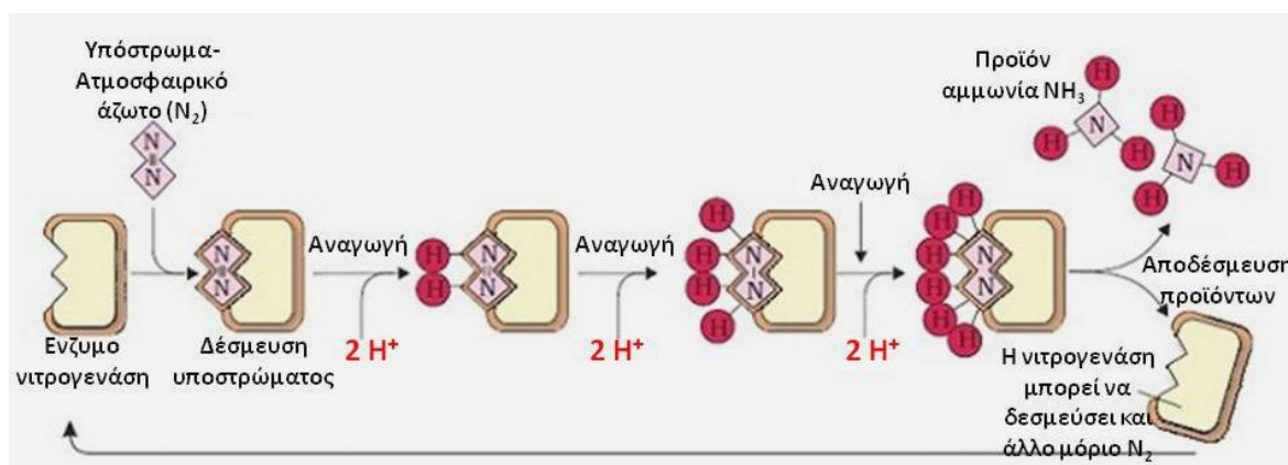
Σχήμα 3.28. Η καθήλωση του ατμοσφαιρικού αζώτου ( N_2 ) από τη νιτρογενάση και η αναγωγή του σε ενωμένο άζωτο υπό μορφή αμμωνίας ( NH_3 ).
